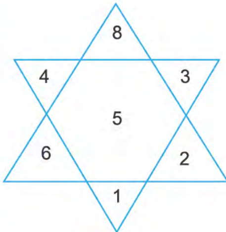
star A
